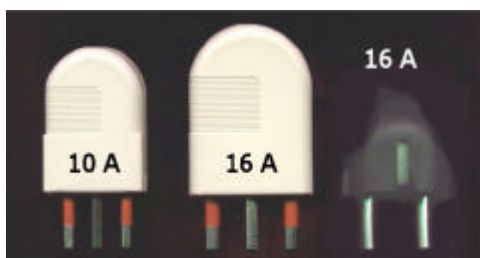
Figura 1. Spine da 10 A, 16 A e Tipo tedesco..
